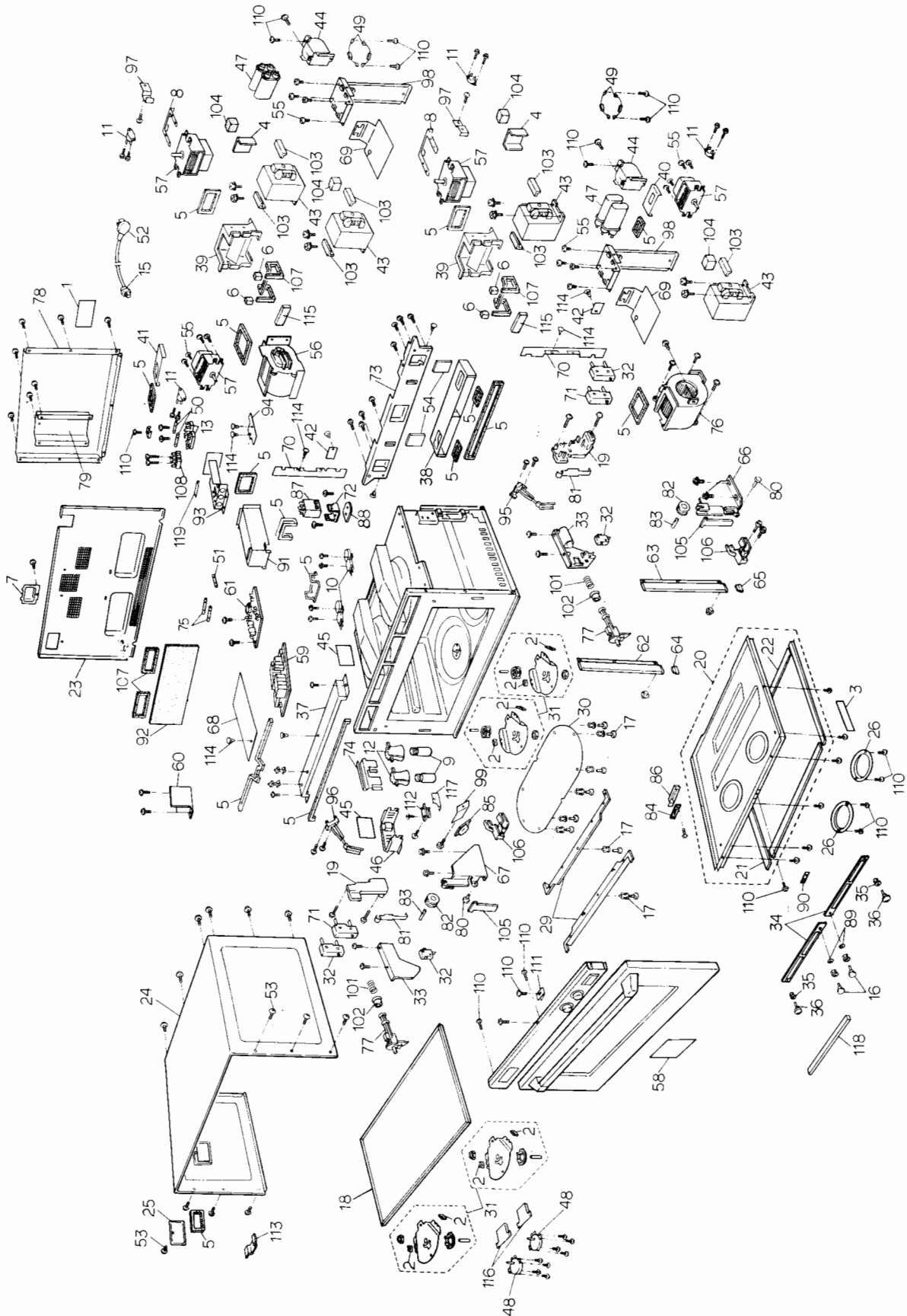
EXPLOSIONSZEICHNUNG (EXPLODED VIEW)
